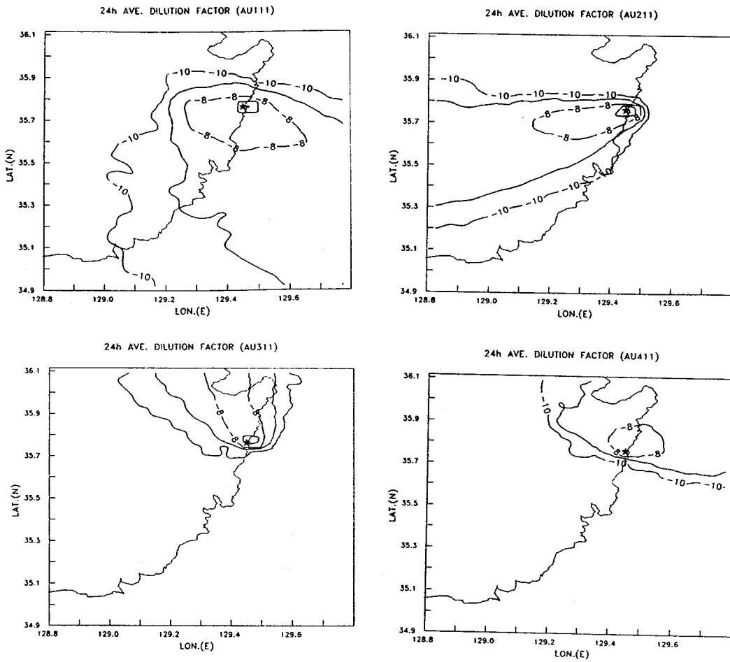
그림 2. 라그랑지안 입자확산 시뮬레이션을 통해 얻어진 일평균 지상 대기확산인자의 분포. 등치선의 숫자는 상용대수로 단위는 \text{sec}/m^3 임. 좌측상단부터 오른쪽으로 각각 중관 기상조건이 가을철 111, 211, 311 그리고 411의 경우
