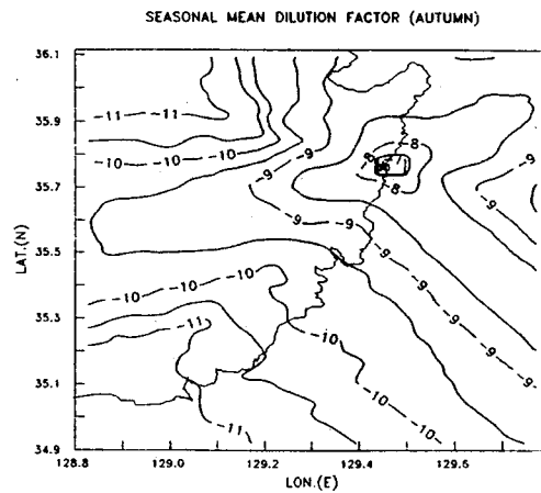
그림 3. 가을철 평균 지상 대기확산인자의 분포. (등치선의 숫자는 상용대수로 단위는 \text{sec}/m^3 임.)
