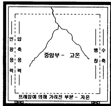
그림 1. Stress distribution in window glass
