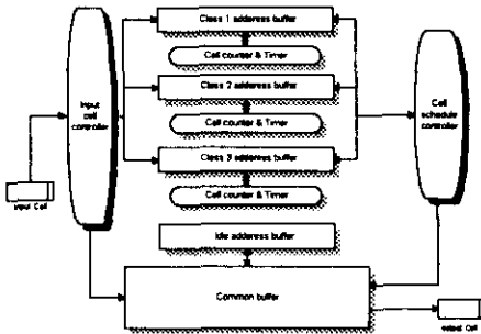
그림 1. 제안된 우선순위 제어 구조
