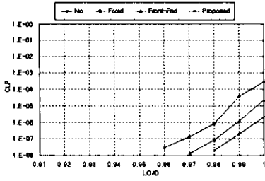
그림 3. Class 1의 셀 손실율
