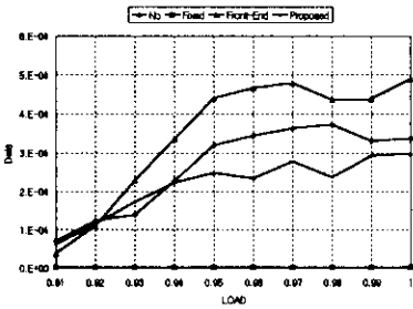
그림 6. Class 1의 셀 지연율
