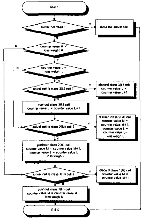
그림 2. 제안된 알고리즘의 흐름도
