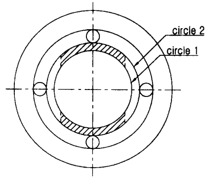
Fig. 4 Noncircular slot
