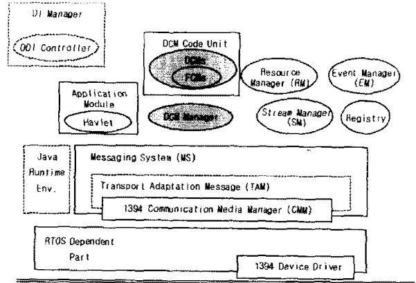
그림 2.1 HAVi FAV (Full AV device)의 구성
