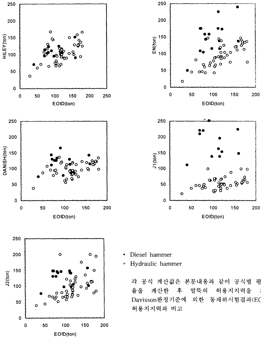
그림 1 각 항타공식에 의한 말뚝지지력과 동재하시험결과(EOID)의 비교
