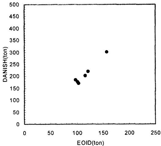
그림 2 A공사 동재하시험결과와 Danish공식의 계산결과 비교
