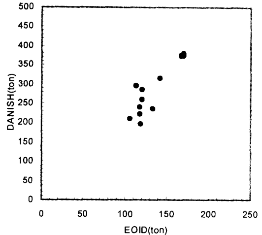
(b) Danish 공식
