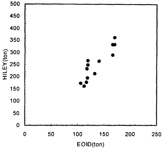
(a) Hiley 공식
