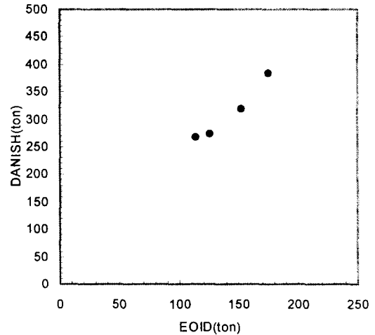
그림 3 B공사 동재하시험결과와 Danish공식의 계산결과 비교
