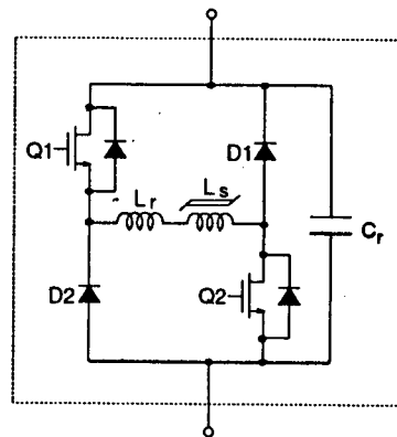
Fig. 1 ZVS PWM module
