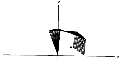
그림 7(a) CASE (ii)에 대한 로봇트 추적 궤적 ( 장애물이 없는 경우 ) Fig. 7(a) The Robot Motion for the CASE (ii). ( without Obstacle )
