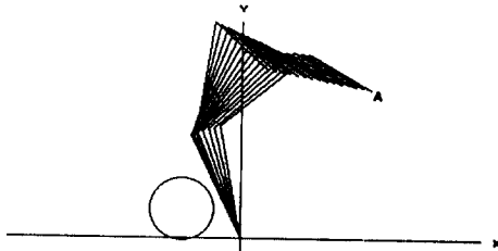
그림 5(b) CASE (i)에 대한 로봇트 추적 궤적 ( 장애물이 있는 경우 ) Fig. 5(b) The Robot Motion for the CASE (i). ( with Obstacle )
