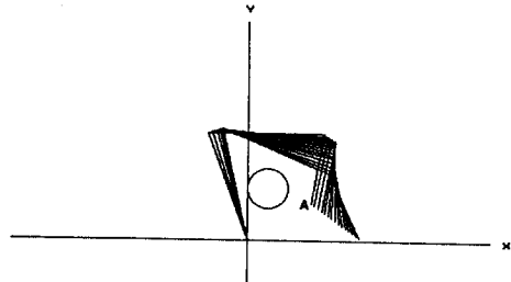
그림 7(b) CASE (ii)에 대한 로봇트 추적 궤적 ( 장애물이 있는 경우 ) Fig. 7(b) The Robot Motion for the CASE (ii). ( with Obstacle )
