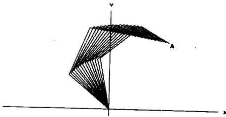
그림 5(a) CASE (i)에 대한 로봇트 추적 궤적 ( 장애물이 없는 경우 ) Fig. 5(a) The Robot Motion for the CASE (i). ( without Obstacle )
