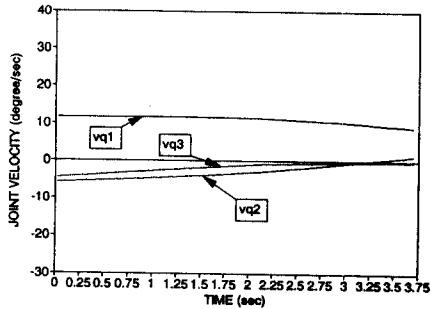
그림 6(a) CASE (i)에 대한 각속도 곡선 ( 장애물이 없는 경우 ) Fig. 6(a) Joint Velocities for the CASE (i) ( without Obstacle )
