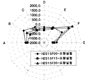
(b) 기반암이 슬래브 천단을 통과(H2)
