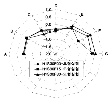
(c) 굴착사면 경사가 30°일 경우
