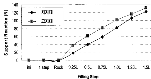
(c) 편경사가 30°일 경우
