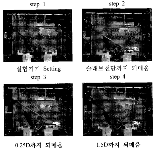
그림 8. 실험수행 과정
