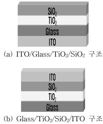
그림 2. 버퍼층 구조. Fig. 2. Buffer layer structure.
