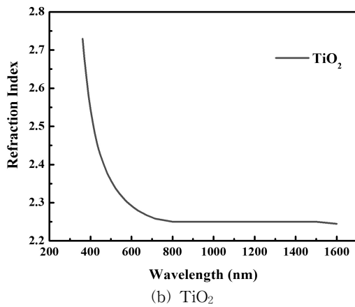
그림 1. Buffer layer 물질의 굴절률. Fig. 1. Index of Buffer layer material.
