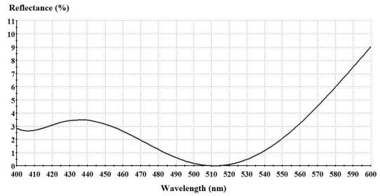
(b) ITO/SiO 2 /TiO 2 /Glass 구조
