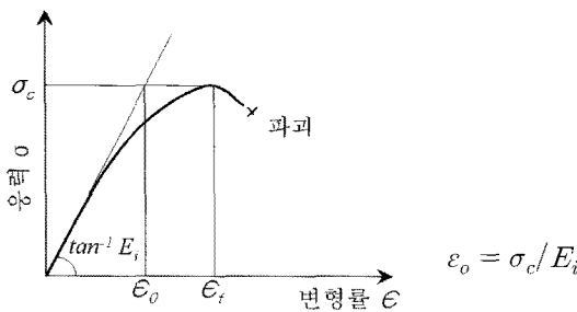
그림 1. 일축압축시험에 의한 응력-변형률도
