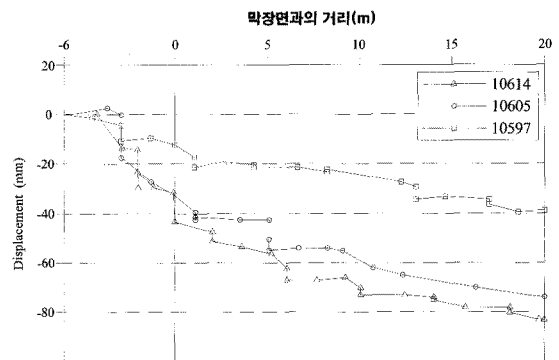
그림 15. S구간의 총변위(선행+계측변위)
