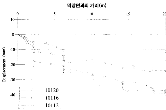
그림 10. 굴착 후 막장면과의 거리에 따른 계측변위(D구간)
