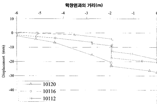
그림 8. 막장과의 거리에 따른 선행변위(D구간)
