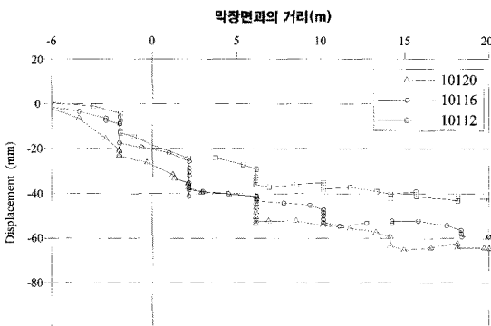
그림 14. D구간의 총변위(선행+계측변위)
