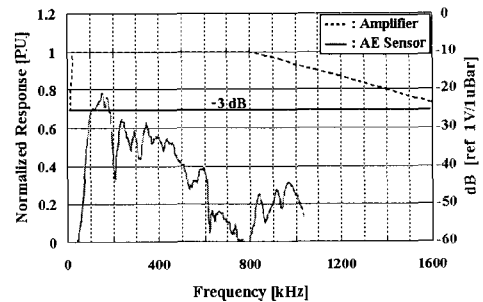
그림 3. 증폭회로의 주파수 응답.
