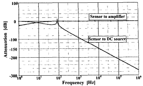
그림 2. 역결합회로의 주파수 응답.
