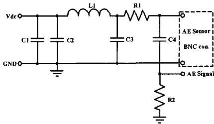
(a) 역결합회로
