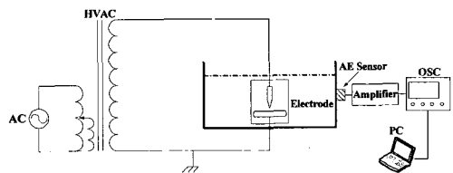
그림 4. 실험장치의 구성.
