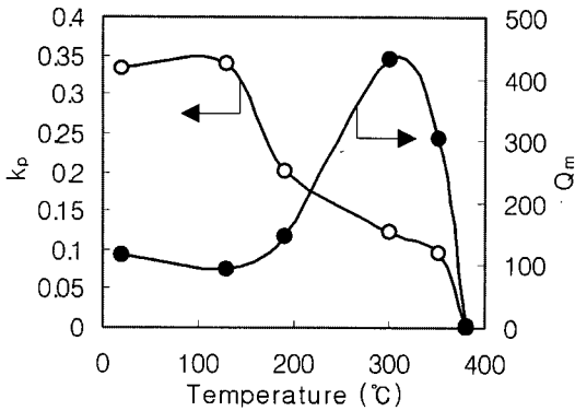
그림 9. CdO=0.02 mol 첨가한 NKN 세라믹스의 k_p 와 Q_m 의 온도의존성.
