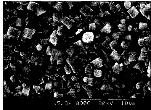
그림 5. CdO=0.015 mol을 첨가한 NKN 세라믹스의 SEM사진. Fig. 5. Microscope of NKN ceramic with addition of CdO=0.015 mol.
