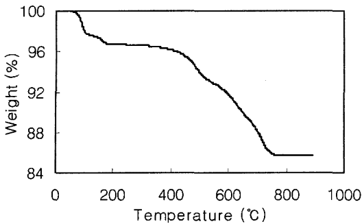
그림 1. NKN 분말의 TGA 곡선.
