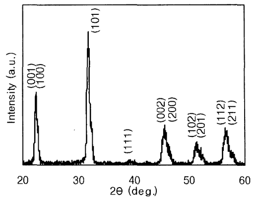
그림 2. 850 °C에서 하소한 분말의 XRD분석.
