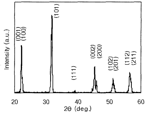
그림 4. CdO=0.03 mol을 첨가한 NKN 세라믹스의 XRD 패턴. Fig. 4. XRD patterns of NKN ceramics with addition of CdO=0.03mol.
