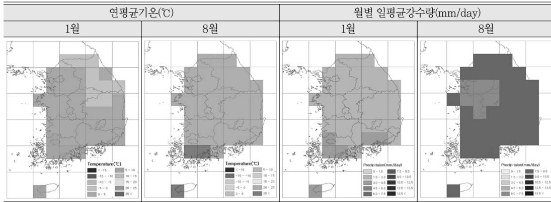
그림 9. RCM으로 추정된 현재기후(1981~1990)
