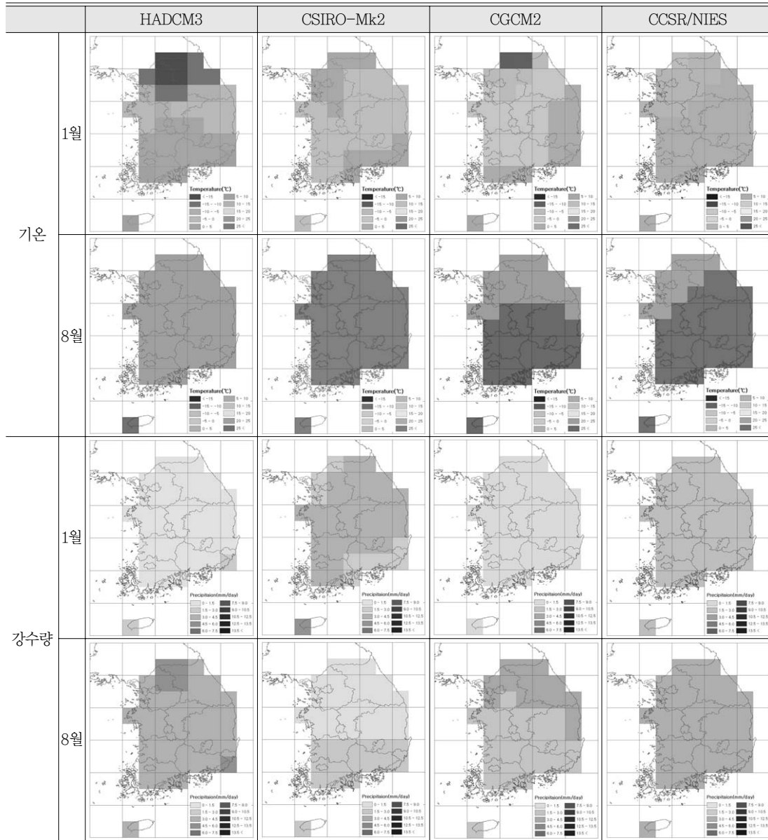
그림 8. GCM으로 추정된 현재기후(1981~1990)
