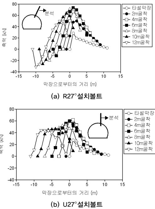
그림 7. 페이스볼트의 설치위치에 따른 축력의 분포 ( \lambda = 1.0D )
