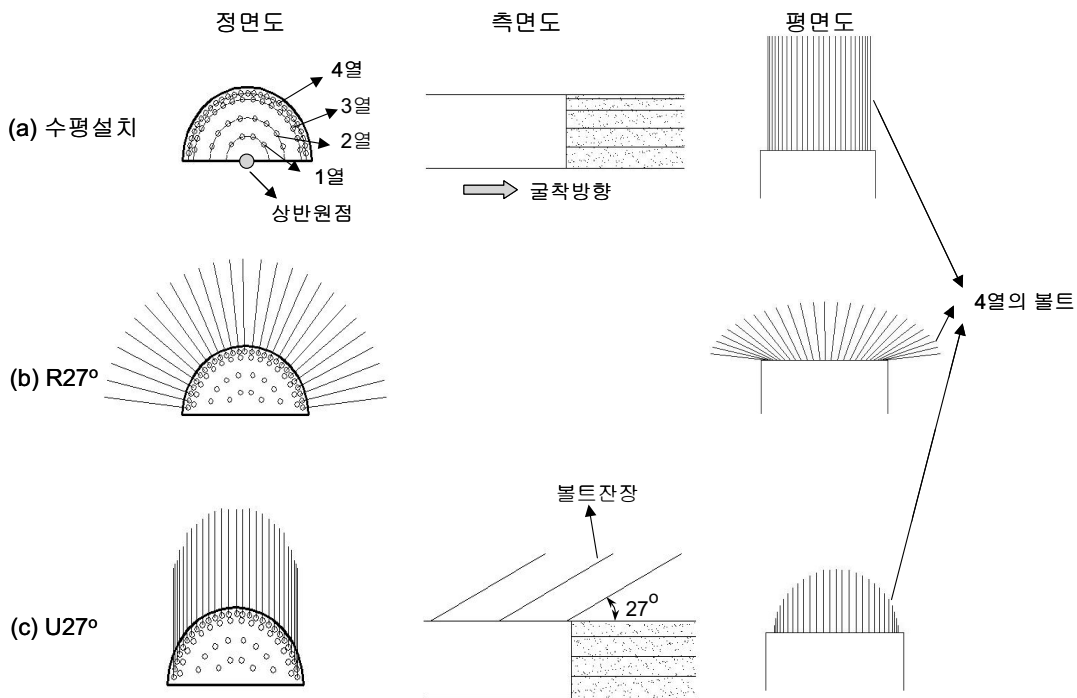
그림 1. 페이스볼트의 설치개념
