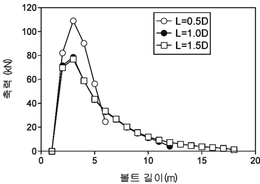
그림 4. 수평설치 볼트의 축력의 크기 비교
