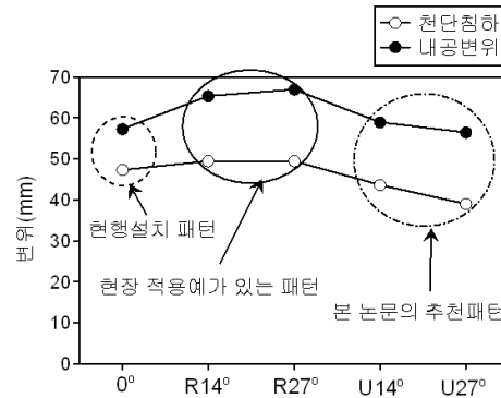
(a) 굴착단면의 변위
