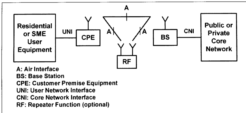
〈그림 6〉 IEEE802.22 WRAN 무선 접속 모델
