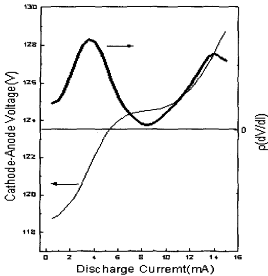
그림 6. Gd/Ne HCD에서 V-I 곡선과 이 곡선의 미분.
