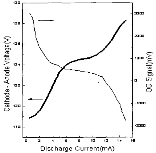
그림 5. Gd/Ne HCD에서 V-I 곡선과 피크 모양 광검류 신호. Fig. 5. The V-I curve and peak-like optogalvanic signals for Gd/Ne HCD.
