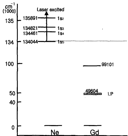
그림 7. Penning 이온화와 관련된 Ne과 Gd의 에너지 준위.
