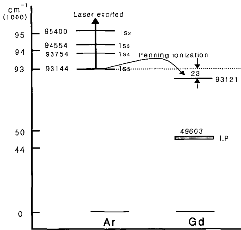
그림 4. Penning 이온화와 관련이 있는 Ar과 Gd의 에너지 준위. Fig. 4. Energy level diagram of Ar-Gd system relevant to the Penning ionization.
