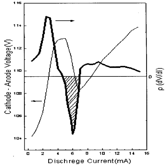
그림 3. Gd/Ar HCD에서 V-I 곡선과 이 곡선의 미분.
