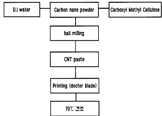
그림 1. CNT 상대전극 제조 공정도.
