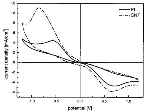
그림 4. CNT 및 Pt 전극에 대한 CV 측정 결과. Fig. 4. Cyclic voltammogram of Pt and CNT. Scan rate was 100 mV/s.
