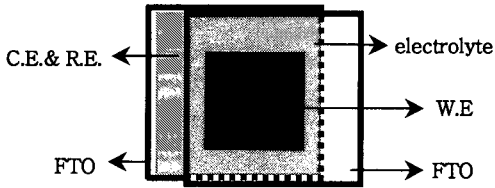
그림 2. 측정용 샘플의 윗면. Fig. 2. Top view of a sample for measurement.
