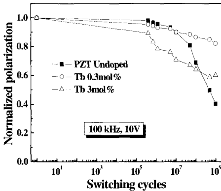
그림 7. Tb 첨가에 따른 PZT 박막의 피로특성. Fig. 7. Fatigue characteristics of PZT thin films as a function of Tb content.
