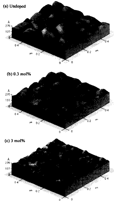
그림 2. Tb 첨가량에 따른 PZT 박막의 AFM 표면 형상.
