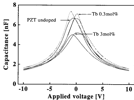
그림 3. Tb 첨가량에 따른 PZT 박막의 C-V 곡선.
