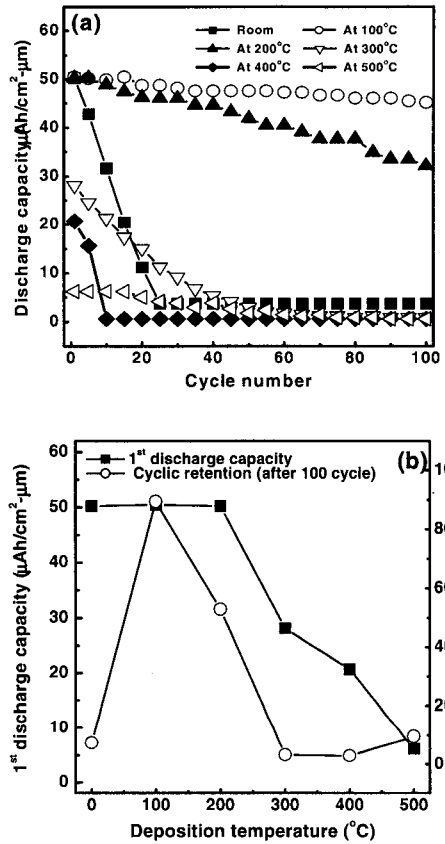
그림 5. 다양한 증착온도에서 증착된 LLTO의 (a) 100 싸이클 동안의 방전용량의 변화와 (b) 초기 방전용량과 싸이클 방전용량 보존률.
