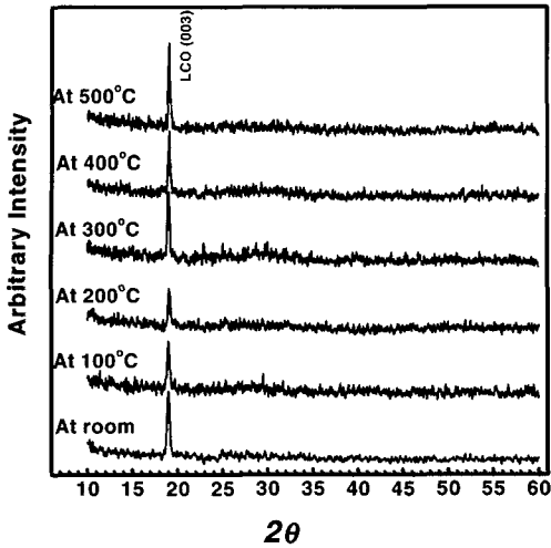
그림 1. 증착온도에 따른 LiCoO 2 /Pt/TiO 2 위에 성장시킨 (Li,La)TiO 3 의 X 선 회절 패턴. Fig. 1. XRD patterns of (Li,La)TiO 3 grown on LiCoO 2 /Pt/TiO 2 substrate at various deposition temperatures.
