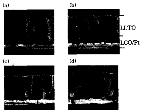
그림 3. 다양한 (a) 상온 (b) 100 °C (c) 300 °C 그리고 (d) 500 °C의 증착온도에 LiCoO 2 /Pt/TiO 2 위에 성장 시킨 (Li,La) TiO 3 의 단면 사진. Fig. 3. Cross-sectional images of LLTO/LCO/Pt/TiO 2 thin films deposited at (a) room, (b) 100, (c) 300, and (d) 500 °C.
