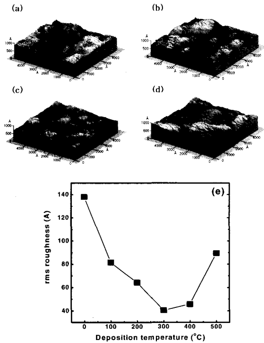
그림 2. 다양한 (a) 상온 (b) 100 °C (c) 300 °C (d) 500 °C의 증착온도에서 LiCoO 2 /Pt/TiO 2 위에 성장시킨 (Li,La)TiO 3 표면 사진, (e) (Li,La)TiO 3 의 표면 거칠기. Fig. 2. Surface morphology of LLTO/LCO/Pt/TiO 2 thin films deposited at (a) room (b) 100 °C (c) 300 °C (d) 500 °C and (e) rms roughness of LLTO.
