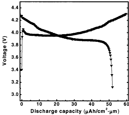
그림 4. 500 °C에서 증착된 LiCoO 2 정극의 충·방전 용량 그래프.
