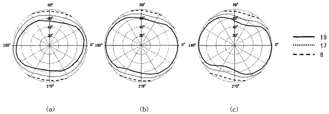
그림 6. R_{100} 일 때 등 반사율 곡선: (a) \lambda=480\text{nm} , (b) \lambda=550\text{nm} , (c) \lambda=630\text{nm} . Fig. 6. Iso-reflectance contour at R_{100} : (a) \lambda=480\text{nm} , (b) \lambda=550\text{nm} , (c) \lambda=630\text{nm} .
