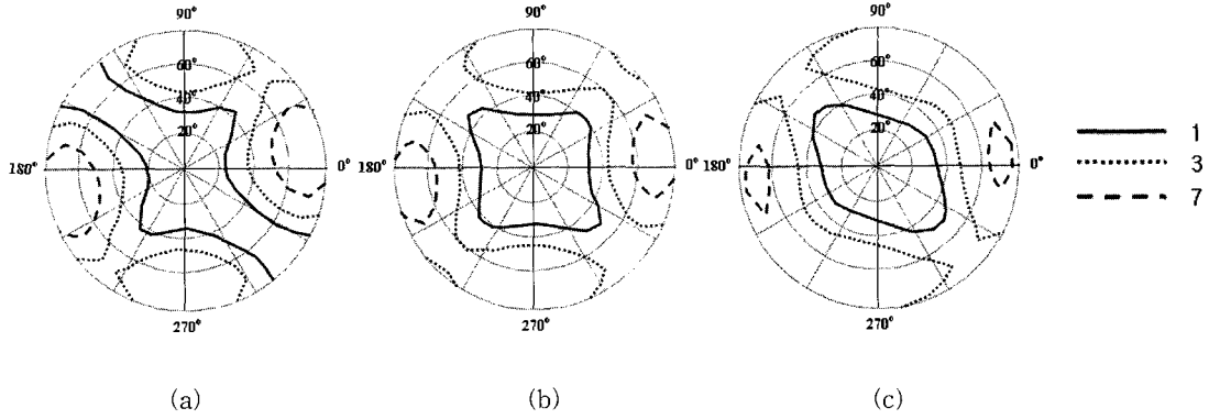
그림 4. R_0 일 때 등 반사율 곡선: (a) \lambda=480\text{nm} , (b) \lambda=550\text{nm} , (c) \lambda=630\text{nm} . Fig. 4. Iso-reflectance contour at R_0 : (a) \lambda=480\text{nm} , (b) \lambda=550\text{nm} , (c) \lambda=630\text{nm} .
