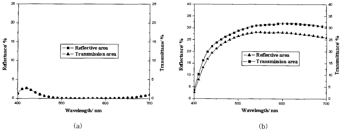
그림 3. 입사 파장에 따른 빛샘 정도: (a) 전압 무인가시, (b) 전압 인가시. Fig. 3. Wavelength dependent-light leakage: (a) off-state, (b) on-state.
