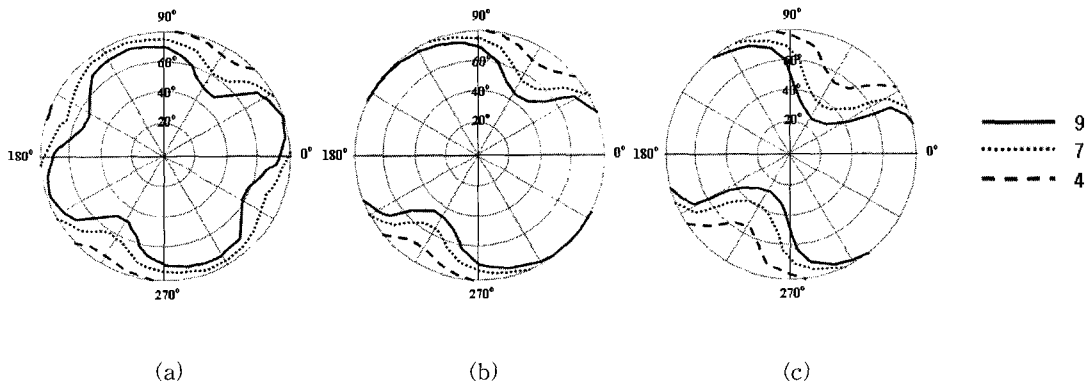
그림 5. R_{50} 일 때 등 반사율 곡선: (a) \lambda=480\text{nm} , (b) \lambda=550\text{nm} , (c) \lambda=630\text{nm} . Fig. 5. Iso-reflectance contour at R_{50} : (a) \lambda=480\text{nm} , (b) \lambda=550\text{nm} , (c) \lambda=630\text{nm} .
