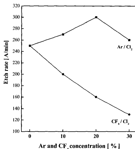
그림 2. Ar/ Cl_2 및 CF_4/Cl_2 가스혼합비에 따른 YMnO_3 박막의 식각속도.
