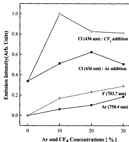
그림 1. Ar/ Cl_2 및 CF_4/Cl_2 가스혼합비에 따른 Ar 이온, Cl 라디칼, F 라디칼의 광 방출 세기.
