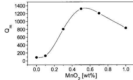
그림 5. MnO 2 첨가량에 따른 기계적 품질계수 (Q m ). Fig. 5. Mechanical quality factor(Q m ) as a function of MnO 2 addition.
