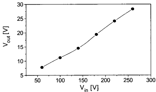
그림 6. 입력전압에 따른 출력전압. Fig. 6. Output voltage as a function of the input voltage.
