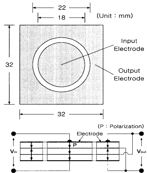
그림 1. 제작된 압전 트랜스포머의 구조.
