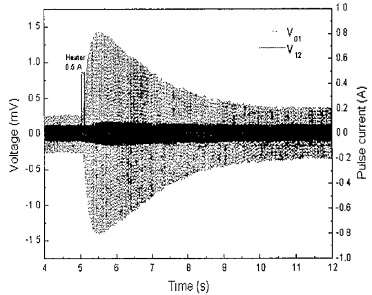
그림 5. 60 K에서 히트펄스에 의한 교류 전압 특성 Fig. 5. AC voltage responses after heat pulse at 60 K.
