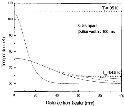
그림 9. 60 K에서 히터펄스에 의한 테이프 길이 방향의 온도 분포. Fig. 9. Temperature(longitudinal direction) traces in tape after heat pulse at 60 K.
