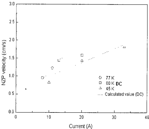
그림 10. 각 온도에서 직류 동작전류에 대한 NZP 속도. Fig. 10. NZP velocity vs DC operating current at each temperature.
