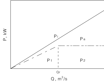
[그림 1] 소수력발전소의 출력특성
