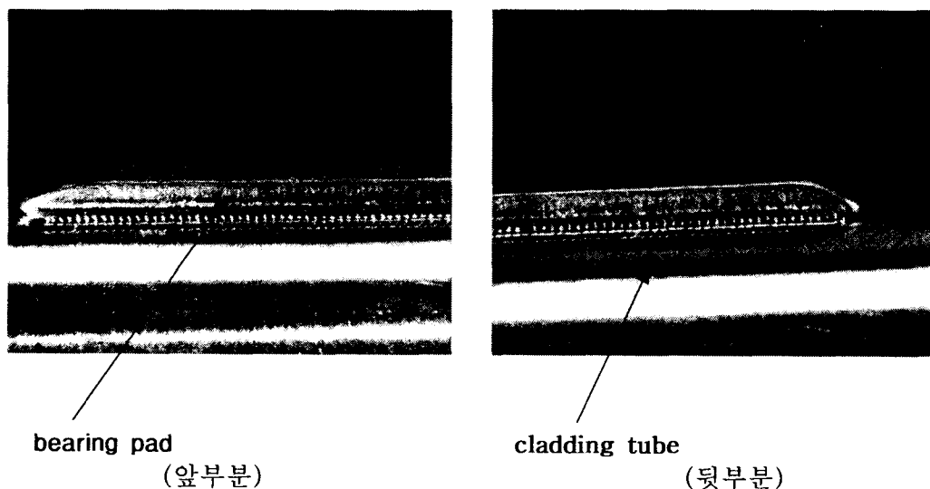
Fig. 1 레이저용접된 피복관과 지지체의 연결부분 (X8)
