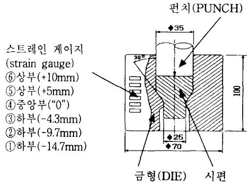
그림 2 전방압출 실험용 금형
