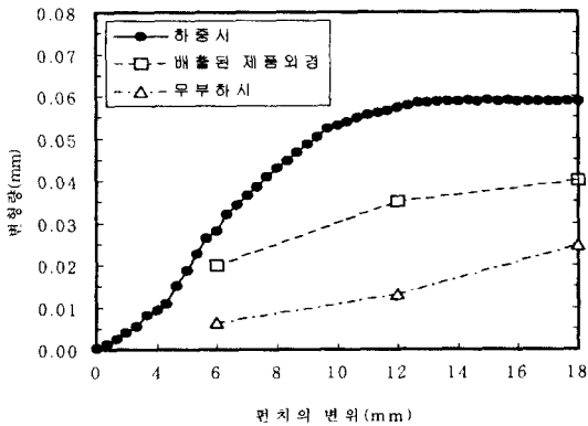
그림 9 컨테이너 중앙부의 금형(⑤번 측정부) 과 제품 변형량 (시편 \phi 35 )
