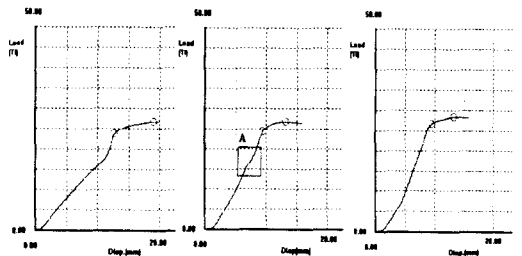
(a) 시험편 \phi 32 \times 34 (b) 시험편 \phi 34.5 \times 30 (c) 시험편 \phi 35 \times 36
