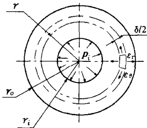
그림 1 금형의 탄성변형
