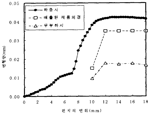
그림 8 컨테이너 중앙부의 금형(⑤번 측정부) 과 제품 변형량 (시편 \phi 34.5 )
