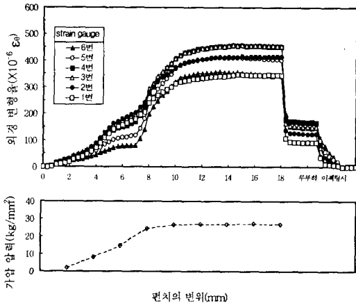
그림 4 편치의 변위에 따른 외경 변형률 (시편 \phi 34.5 )
