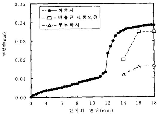
그림 7 컨테이너 중앙부의 금형(⑤번 측정부) 과 제품 변형량 (시편 \phi 32 )
