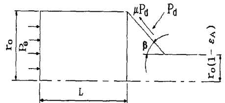
그림 6 전방압출에 있어서 경사금형 부분의 내압
