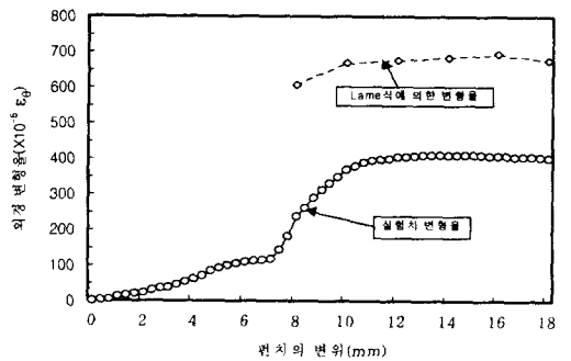
(a) 컨테이너 금형부분(⑤번 측정부)
